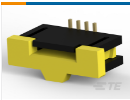
TE Part # 1734248-4 1.0 FPC, ZIF V/T, SMT, 4P
